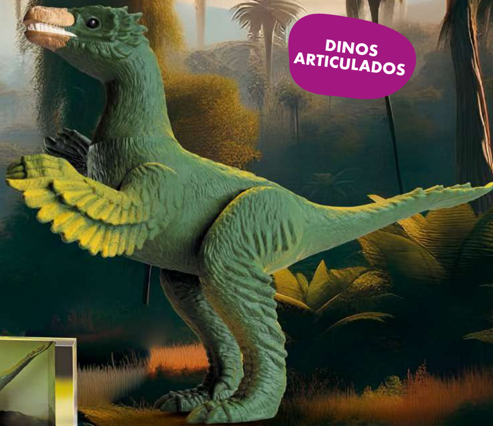
Deinonychus
